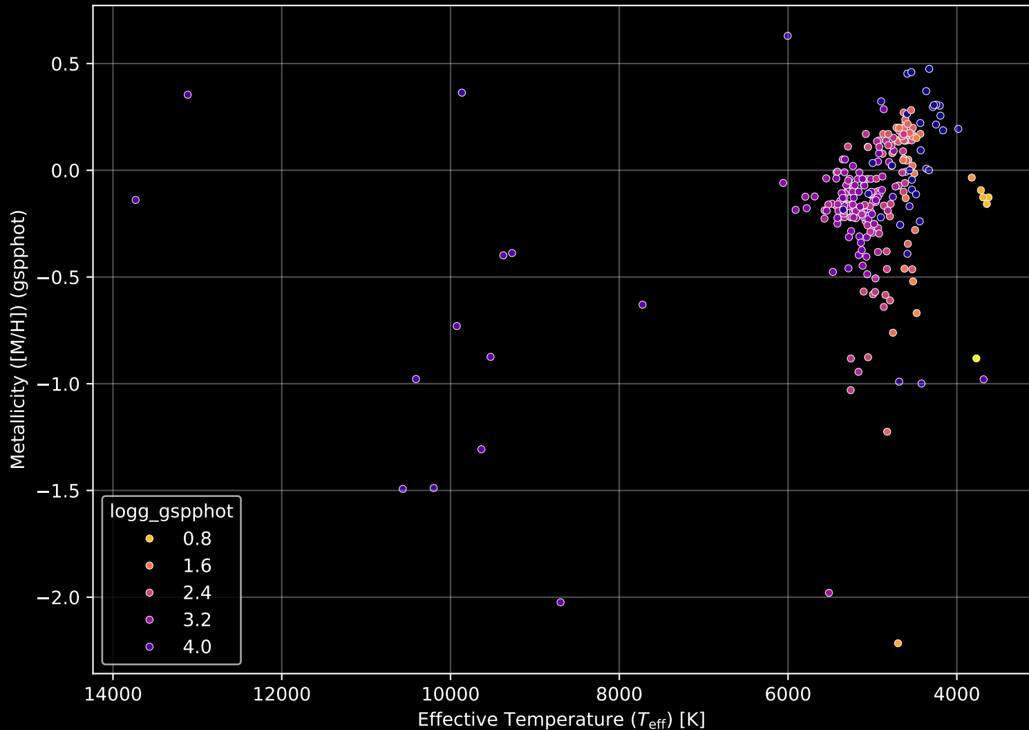
APOGEE DR17 Field: [Berkeley_22_btx] Stellar Population Parameters (n= 263)
